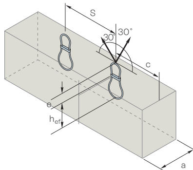
Longitudinal Installation
